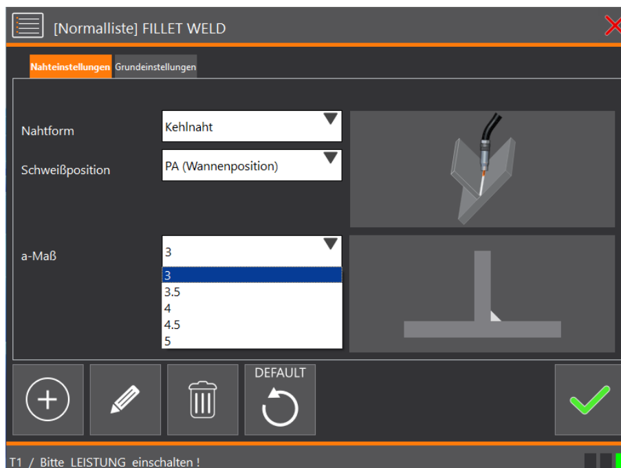
Bild 1: QIROX Easy Weld unterstützt Anwender bei der Erstellung von Schweißparameterlisten.
